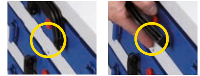
Schubladen-Einzelverriegelung verhindert selbstständiges Öffnen
